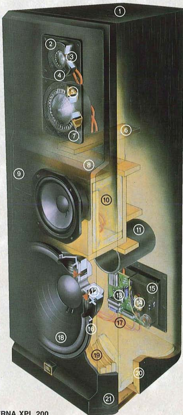
VISTA INTERNA XPL 200
